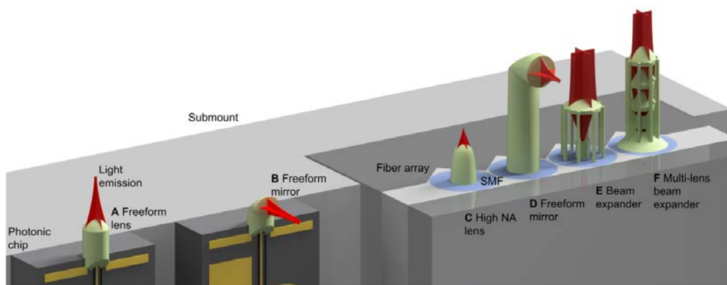
Bild 2: Strahlformende Elemente (hellgrün) werden durch dreidimensional-direkt-schreibende Nanolithographie in-situ an den Facetten photonischer Komponenten hergestellt. (Quelle: KIT/Vanguard Photonics)
