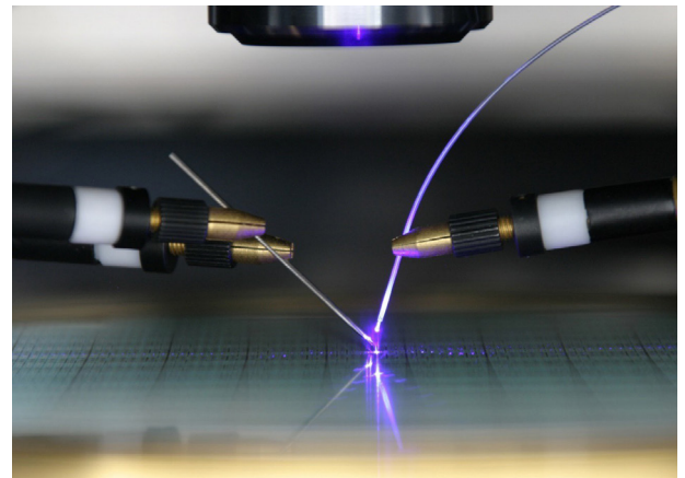
Charakterisierung von neuen optoelektronischen Sensoren im Waferverbund.
