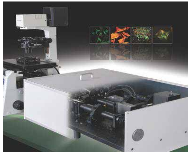
Bild 2: Einzelmolekülsensitives, konfokales Fluoreszenz-Lebensdauer-Mikroskop (Quelle: PicoQuant GmbH, Berlin)
