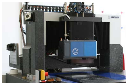
Bild 2: X-Y-Z-Gantry mit montiertem 3-Achs-Galvanometer-Scanner (Quelle: ARGES GmbH)
