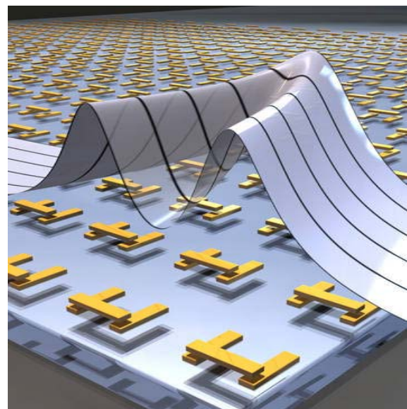
Photonische Metamaterialien (Quelle: Uni Stuttgart)
