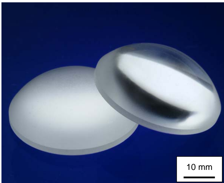
Unbehandelte (links) und laserpolierte Glaslinse (rechts)
